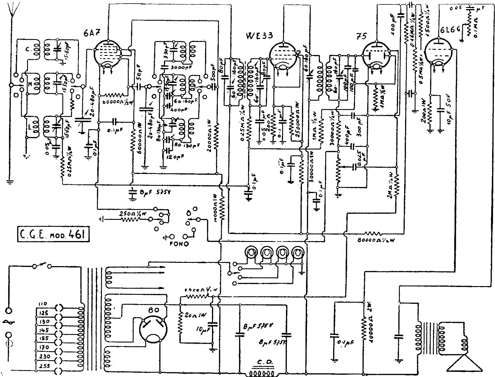
COMPAGNIA GENERALE DI ELETTRICITÀ. — Modello « 461 ». - Produzione 1938. - Media frequenza: 459 kHz.
